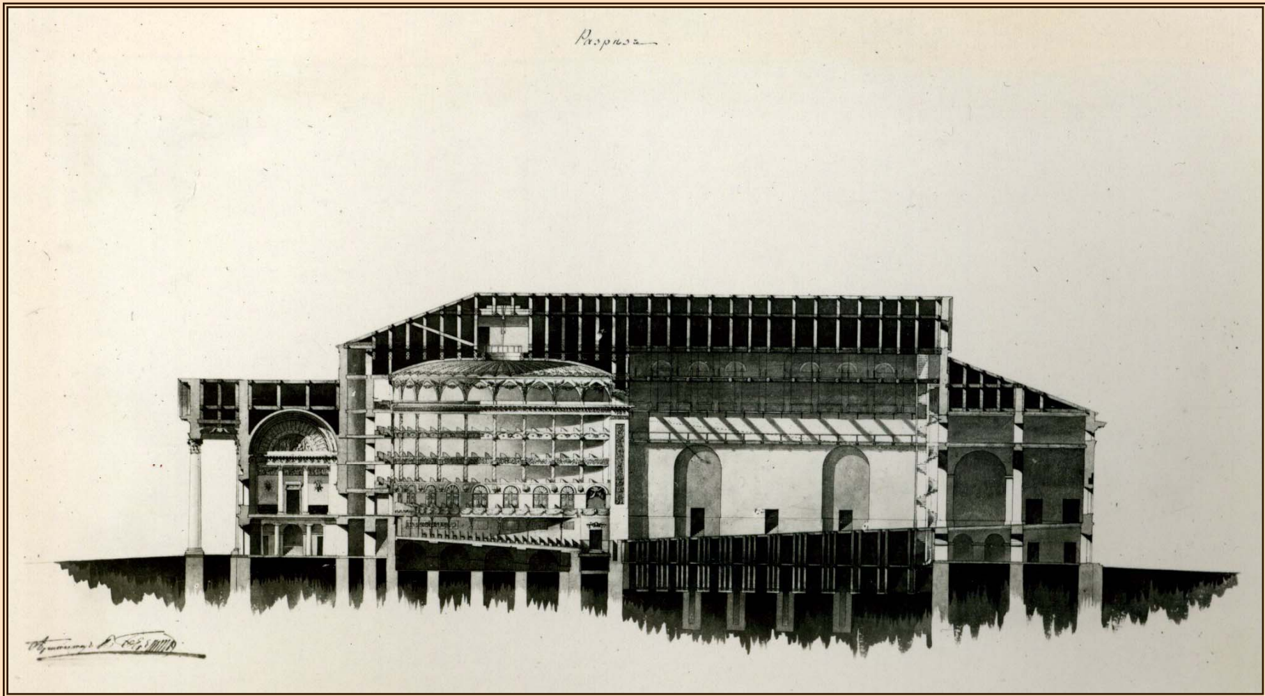
Проект міського театру. Поздовжній розріз. Автор В.І. Беретті, б/д. Копія. ЦДАМЛМ України. Ф. 236, оп.1, од.зб. 3, арк. 205
